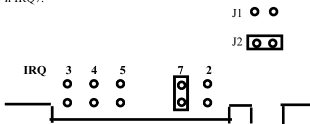
рис.1 Установка переключателя вектора прерывания (пример: IRQ7, баз. адрес 180H)
